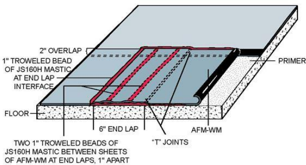
END LAP/T-JOINT
